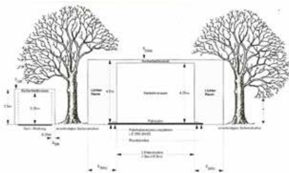
S_0 = seitlicher Sicherheitsraum S_0 = oberer Sicherheitsraum R = Radfahrer Kfz = Kraftfahrzeug * Kronenansatz in Abhängigkeit von Baumart, Wuchstform des Baumes, angrenzende Nutzung und Topographie (z. B. bei Einreihung)
